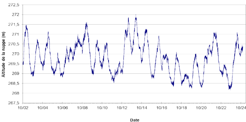
Piézomètre de Villars-les-Dombes Niveau piézométrique du 17 octobre 2002 au 18 décembre 2024
